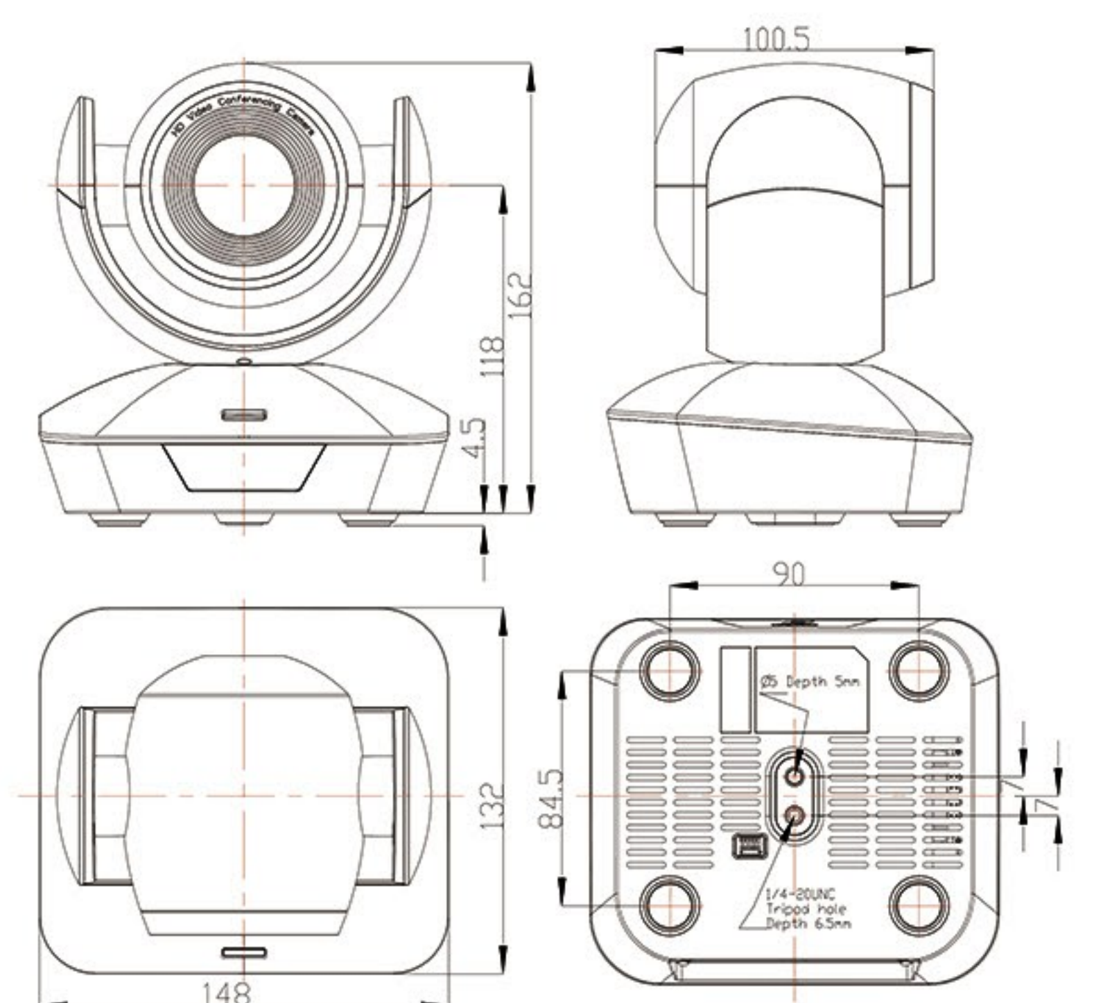
尺寸图(毫米)
