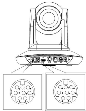
VISCA IN 与 Mini DIN 接线表
