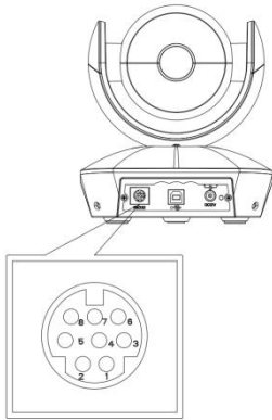
VISCA IN 与 DB9 接线表
