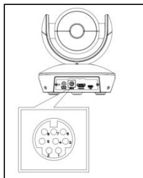
VISCA IN 与 Mini DIN 接线表
