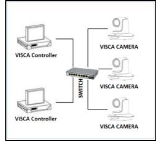
IP 组网方式
