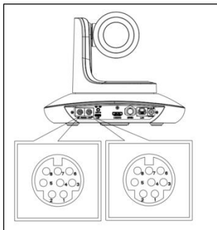
VISCA IN 与 Mini DIN 接线表
